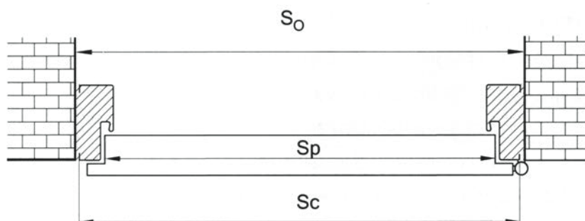
Sposób wymiarowania drzwi z ościeżnicą „11” oraz TERMO
