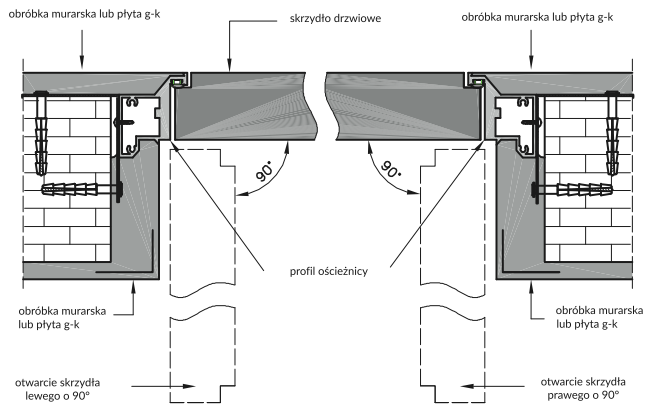
Przekrój poprzeczny drzwi Sara Eco 2
