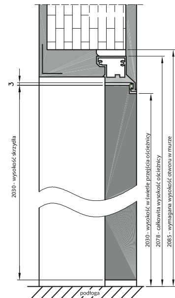
Przekrój pionowy drzwi Sara Eco 2
