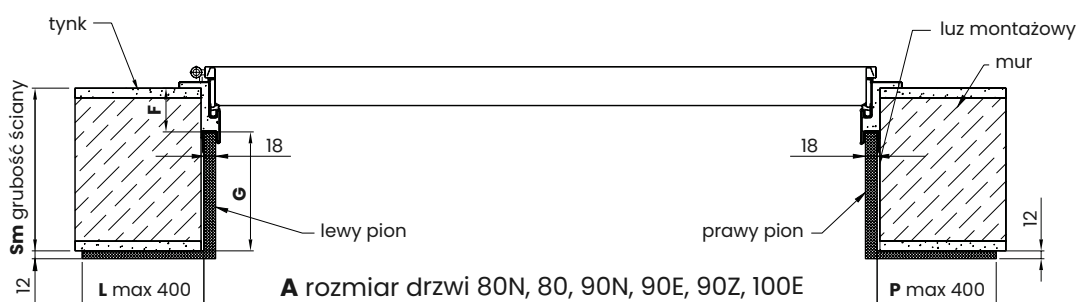
PRZEKRÓJ POZIOMY
