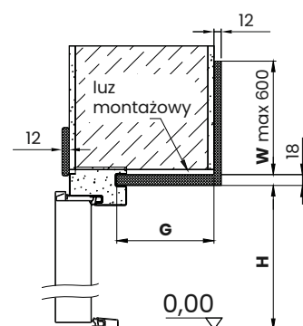
PRZEKRÓJ PIONOWY
