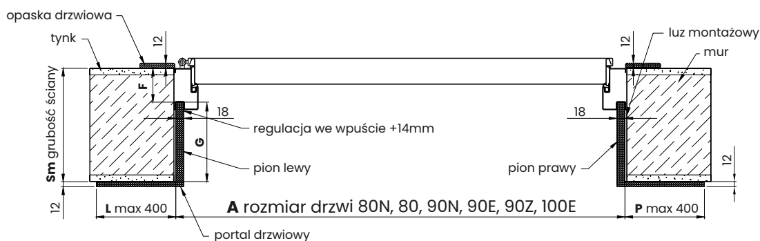
PRZEKRÓJ POZIOMY
