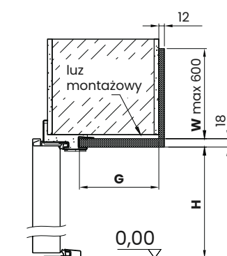
PRZEKRÓJ PIONOWY
